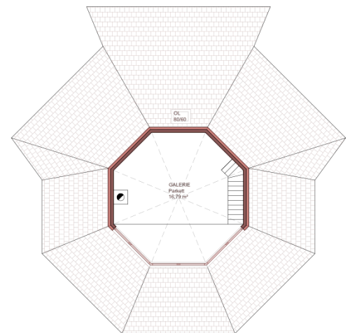
GRUNDRISS OG 1:100
