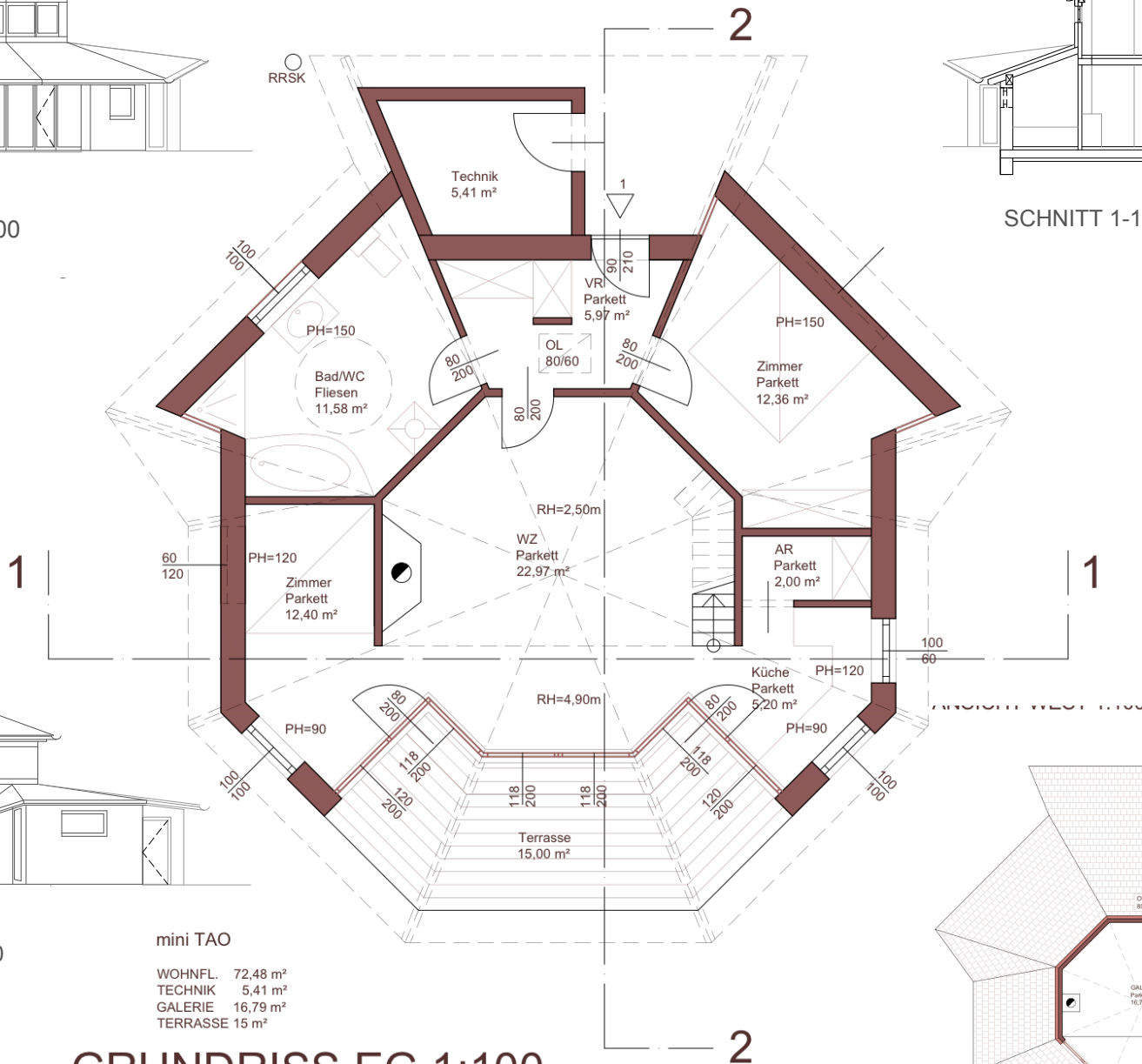
GRUNDRISS EG 1:100
