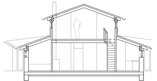
SCHNITT 1-1 1:100
