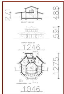
ANSICHT SÜD 1:100
